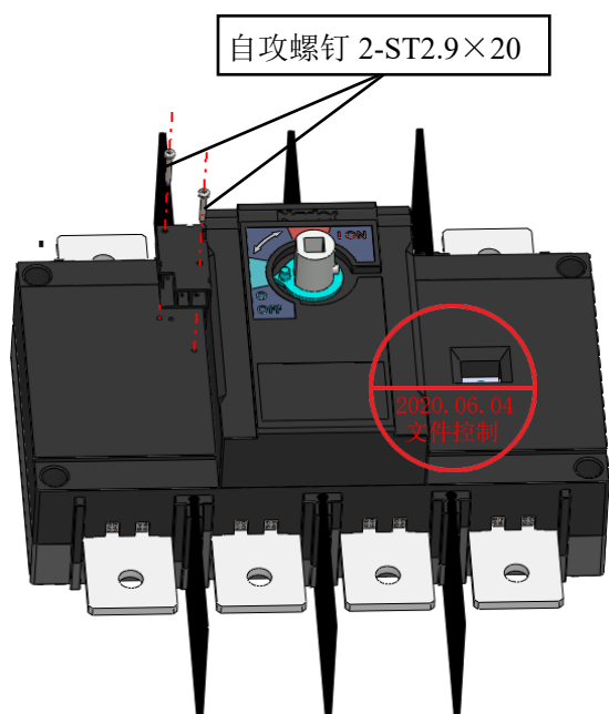
辅助触头安装 (一个)
