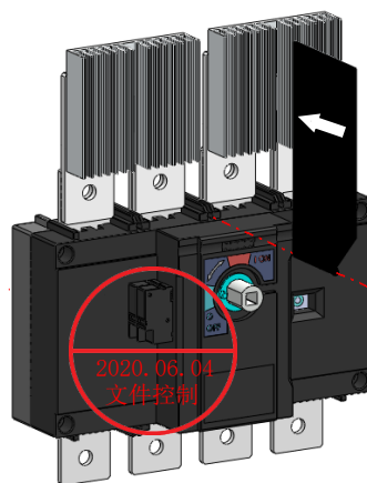
带短接排产品相间隔板安装
