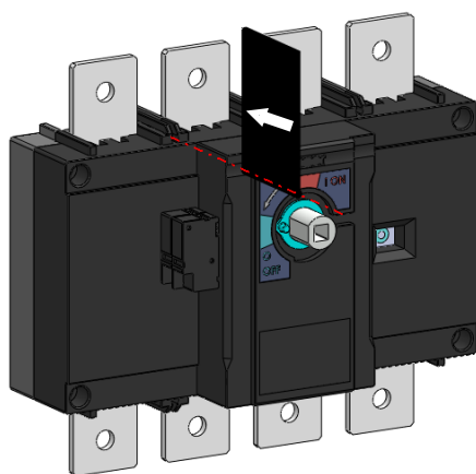
基本型产品相间隔板安装
