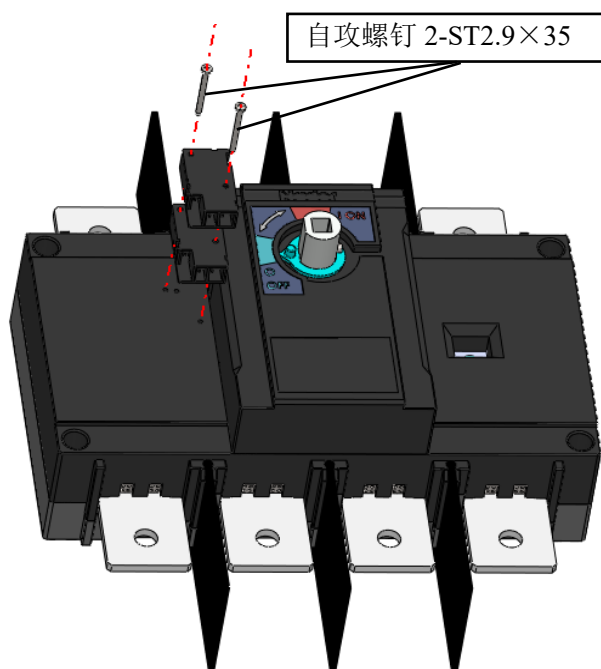
辅助触头安装 (二个)
